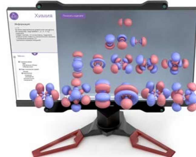
Атомные орбитали
