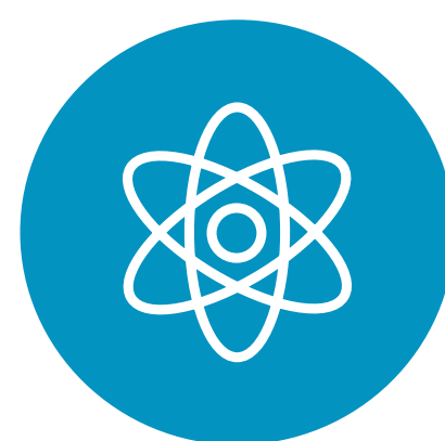
Физика
