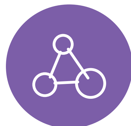
Химия
