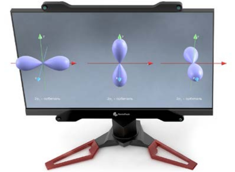
2-й энергетический уровень
