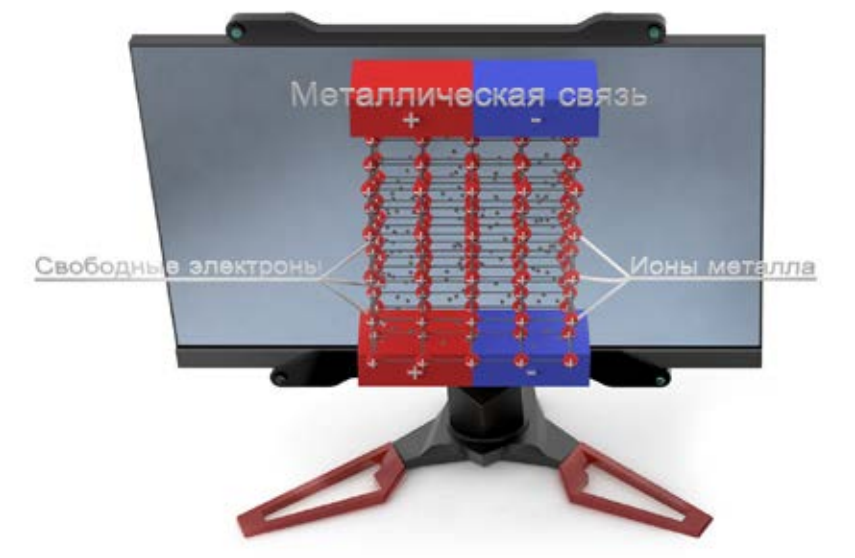
Металлическая связь
