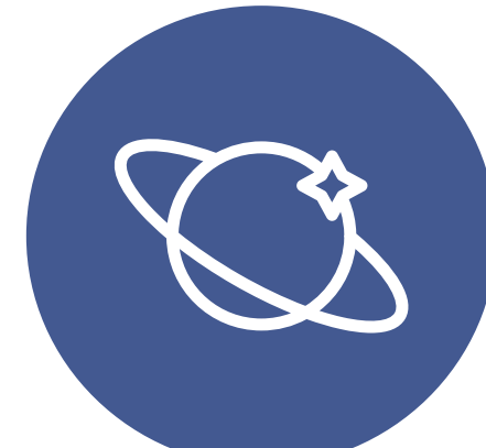
Астрономия
